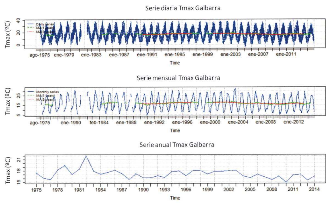
Representación gráfica de las series de datos de temperatura máxima de las series de Galbarra, Iguzquiza y Larraona.
