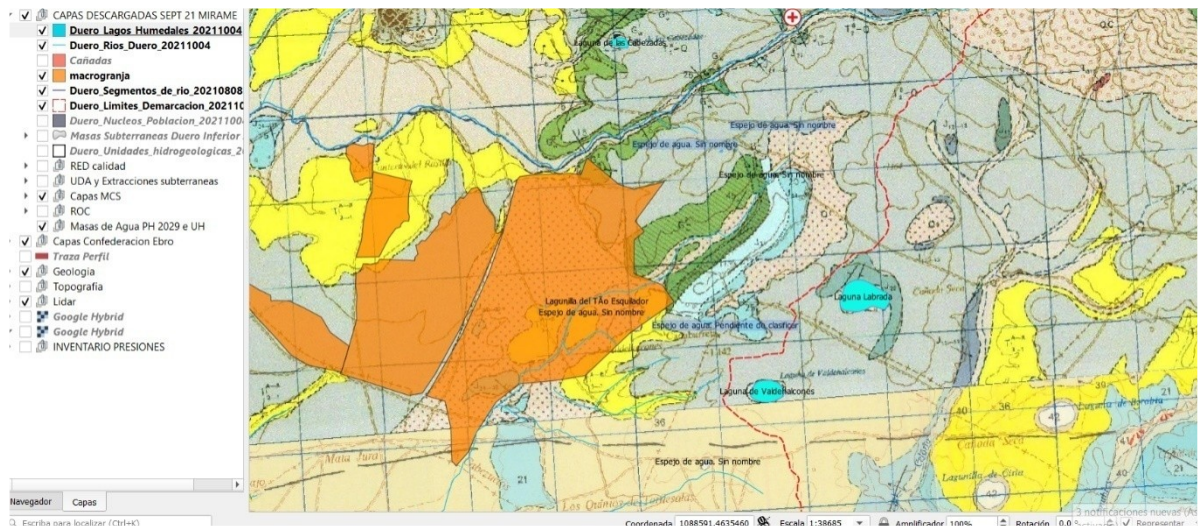
Figura 2: Mapa geológico de la zona de Noviercas. Hoja 351 Noviercas y Hoja 380 Borobia. 2ª Serie Magna. IGME. En colores azules calizas jurásicas, por debajo de cuaternarios y terciarios en colores grises y amarillos. En naranja el emplazamiento previsto para la granja.
