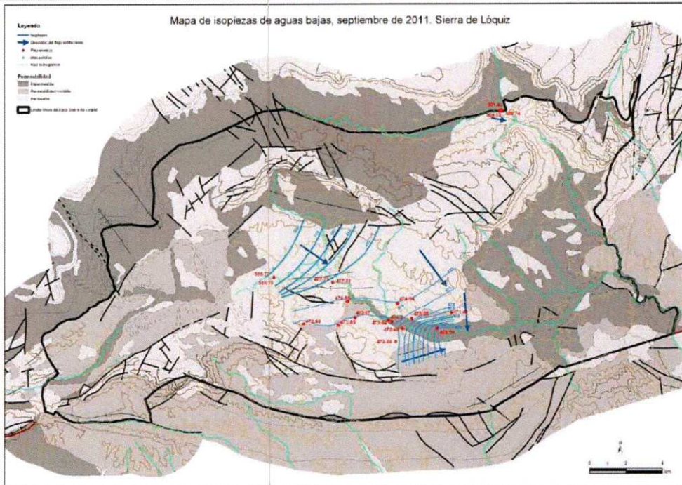
Figura 20: Mapas de piezometría (aguas bajas y altas) de la Sierra de Lóquiz en los últimos años. Fuente: web del Gobierno de Navarra (El Agua en Navarra). Continuación.
