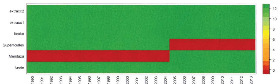
Figura 5: Número de meses con datos válidos para cada año en las series de extracción de agua de la Mancomunidad de Montejoyra. Explicación en el texto.
