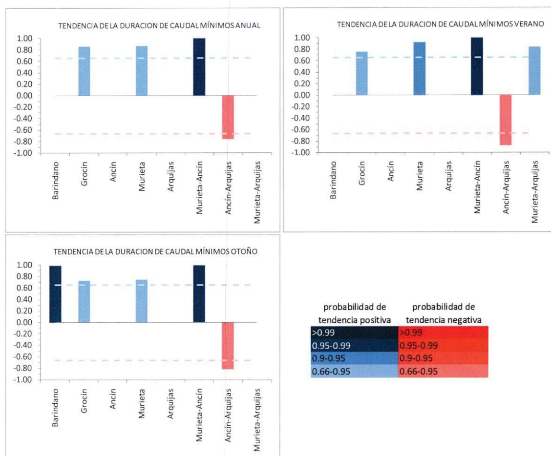
Figura 15: Tendencias de la duración de los caudales menores a Q20 a escala anual y para las estaciones de verano y otoño.
