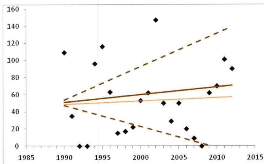
Figura 2: Ejemplo de representación de la pendiente de una tendencia y sus límites superior e inferior. La línea amarilla se refiere a una tendencia lineal de la serie. La línea marrón sólida se refiere a la tendencia lineal obtenida mediante el método de Mann-Kendall. Las líneas discontinuas se refieren a los límites superior e inferior de la banda de confianza de la tendencia obtenida mediante Mann-Kendall.
