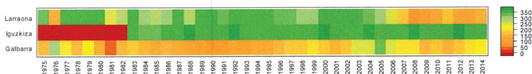
Figura 6: Número de días con datos válidos para cada año en las series de precipitación de las estaciones meteorológicas de Larraona, Iguzkiza y Galbarra.
