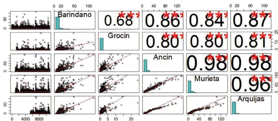
Figura 4: Regresiones y coeficientes de determinación entre las series de caudal analizadas. La primera columna muestra los datos de caudal existentes en cada una de las series. Los gráficos (azul) dispuestos en diagonal muestran los nombres de las estaciones de aforo y los histogramas correspondientes a dichos datos. Los gráficos a la izquierda de esta diagonal se refieren a las regresiones entre cada par de series, y los datos a la derecha de la diagonal a los coeficientes de determinación y la significancia de dichas regresiones. Regresión significativa a nivel: *** = 0.001 ; ** = 0.01 ; * = 0.05 .
