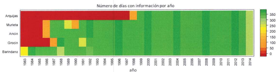
Figura 3: Número de días con datos válidos por año en las series de caudal de Arquijas, Murieta, Ancín, Grocín y Barindano.
