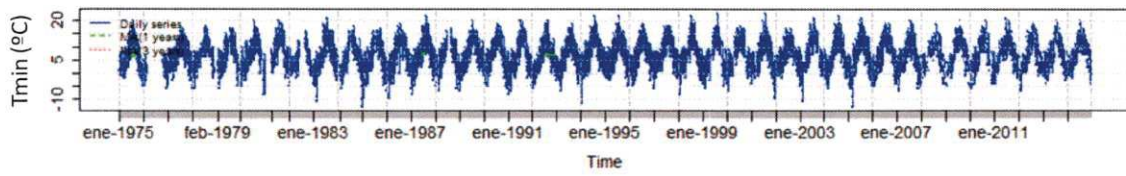
Serie mensual Tmin Larraona
