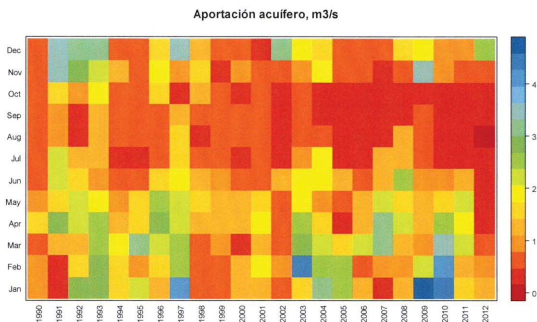
Figura 18: Representación gráfica de la serie de datos de aportación del acuífero al Ega entre Ancín y Murieta a escala mensual para cada uno de los años analizados en este estudio. Los colores rojos indican menores aportes y los azules mayores aportes.
