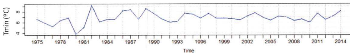
Serie anual Tmin Galbarra
