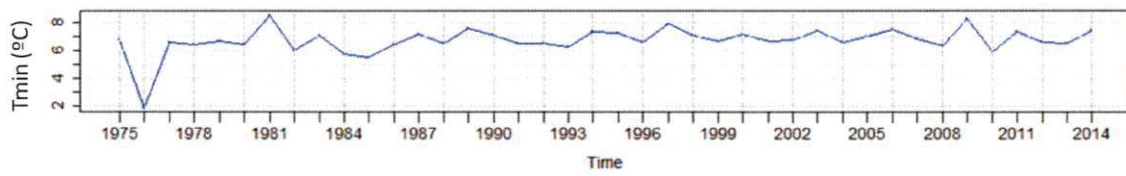
Serie anual Tmin Larraona
