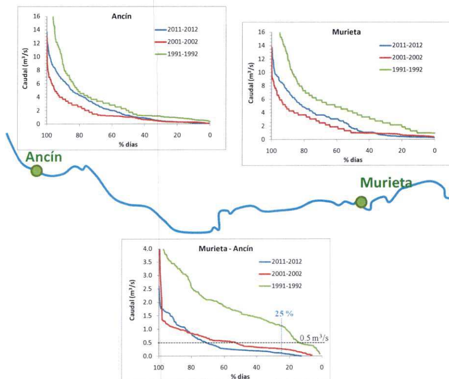
Figura 19: Porcentaje de días con un caudal menor a uno cualquiera a situar en el eje vertical de la gráfica para los años hidrológicos 1991-1992, 2001-2002 y 2011-2012 en las estaciones de aforo de Ancín y Murieta y la serie de caudal que resulta de la resta de ambas series.
