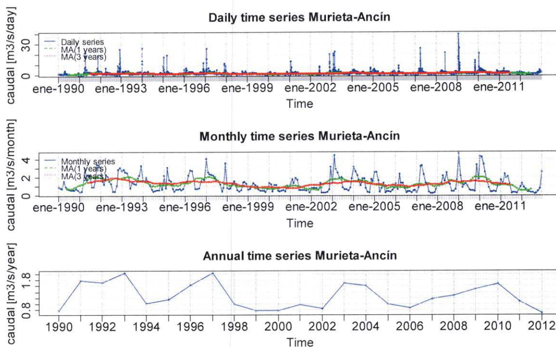
Figura 17: Representación gráfica de la serie de datos de aportación del acuífero al Ega entre Ancín y Murieta a escala diaria, mensual y anual y de las medias móviles de 1 y 3 años.
