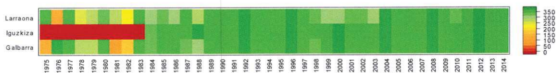
Figura 7: Número de días con datos válidos para cada año en las series de temperatura máxima diaria de las estaciones meteorológicas de Larraona, Iguzkiza y Galbarra.
