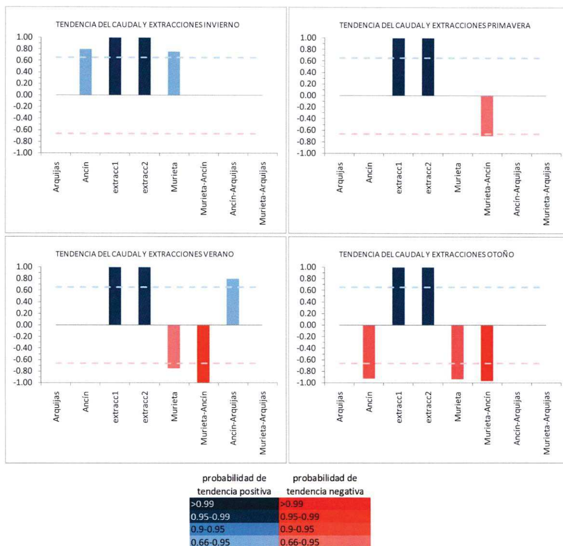
Figura 14: Tendencia estacional de las series de caudal del río Ega y de las extracciones. Solamente se han representado aquellas tendencias con una probabilidad de ocurrencia mayor del 66%.
