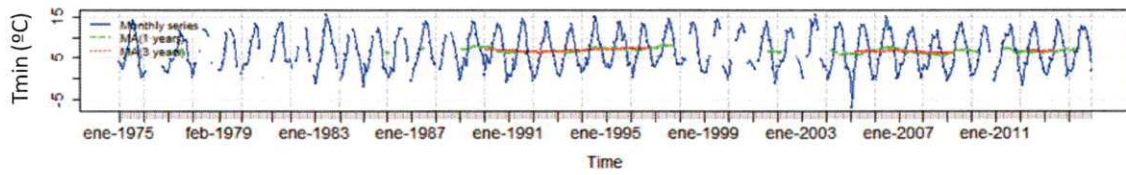
Serie anual Tmin Larraona
