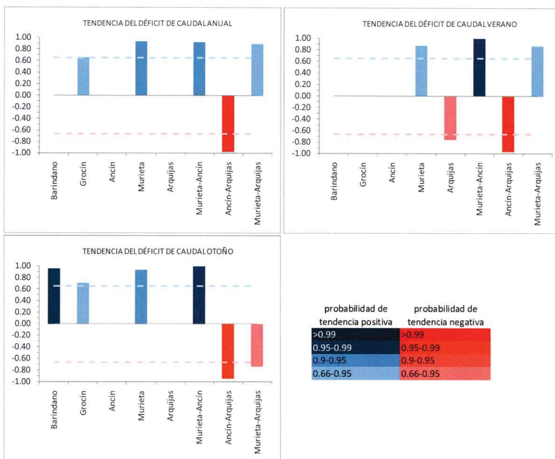
Figura 16: Tendencias del déficit volumétrico de los caudales menores a Q20 a escala anual y para las estaciones de verano y otoño.
