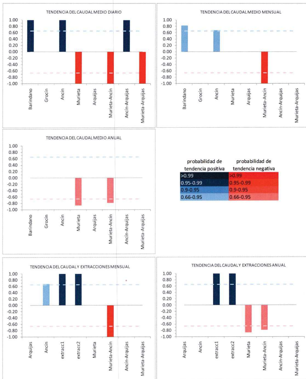
Figura 11: Tendencia de las series de caudal a escala de tiempo diaria, mensual y anual. También se han incluido las tendencias de extracciones junto con las tendencias de caudales del Ega. Solamente se han representado aquellas tendencias con una probabilidad de ocurrencia mayor del 66% ( \pm 0.66 ).
