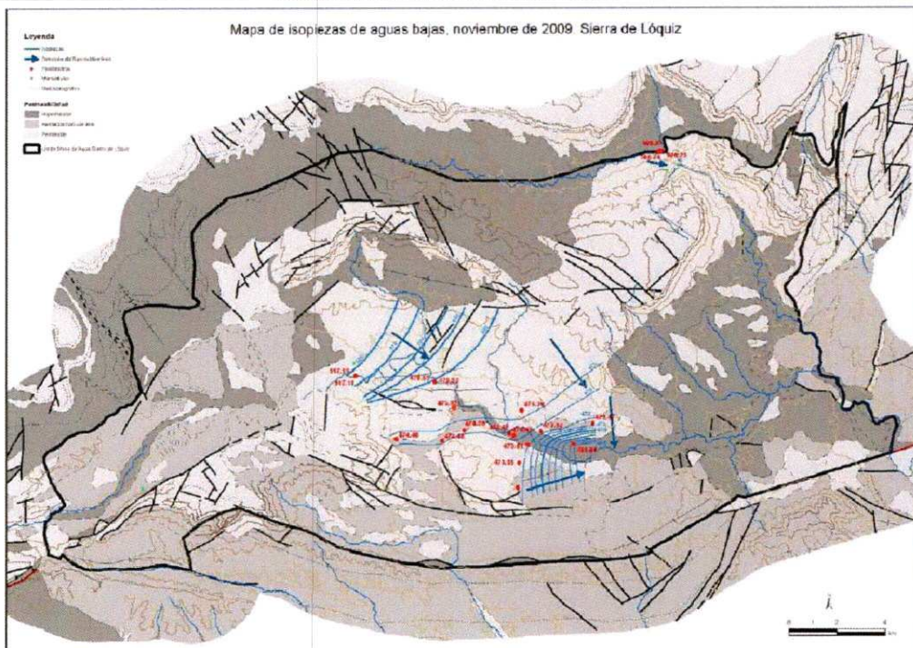
Figura 20: Mapas de piezometría (aguas bajas y altas) de la Sierra de Lóquiz en los últimos años. Fuente: web del Gobierno de Navarra (El Agua en Navarra).
