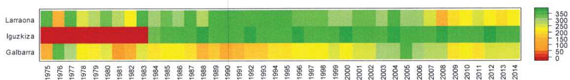
Figura 8: Número de días con datos válidos para cada año en las series de temperatura mínima diaria de las estaciones meteorológicas de Larraona, Iguzkiza y Galbarra.
