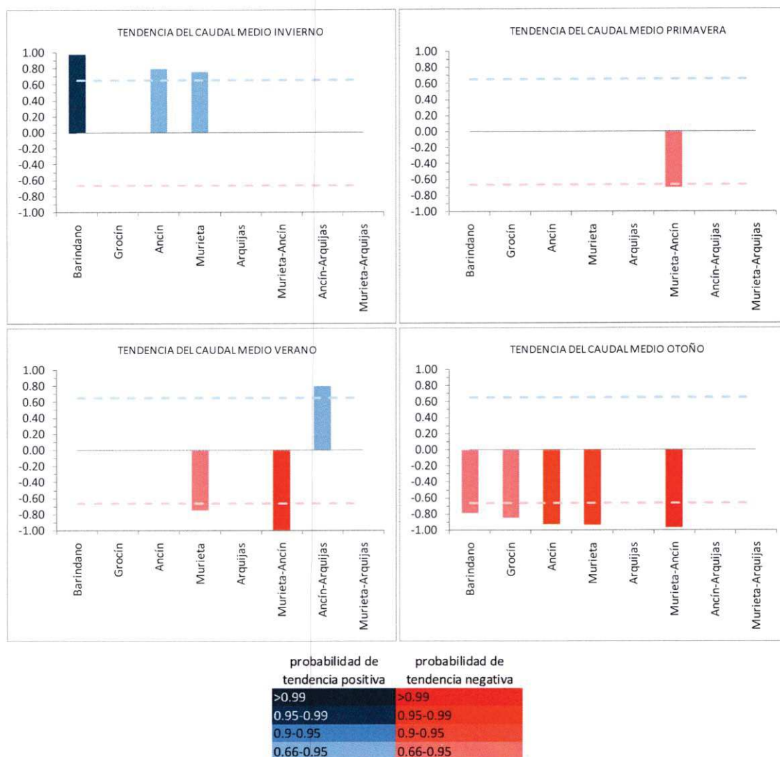
Figura 13: Tendencia de las series de caudal estacional. Solamente se han representado aquellas tendencias con una probabilidad de ocurrencia mayor del 66%.
