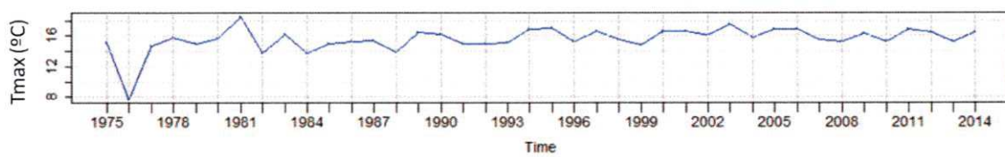
Serie anual Tmax Larraona
