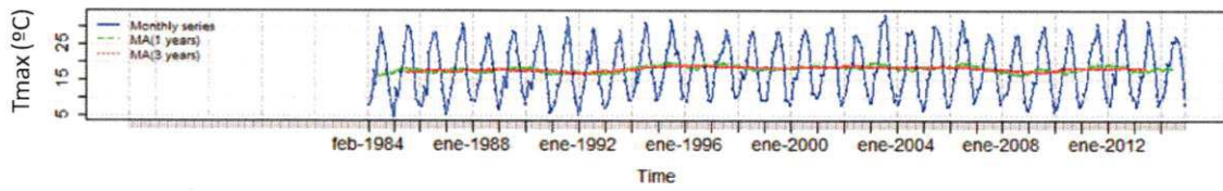
Serie anual Tmax Iguzquiza
