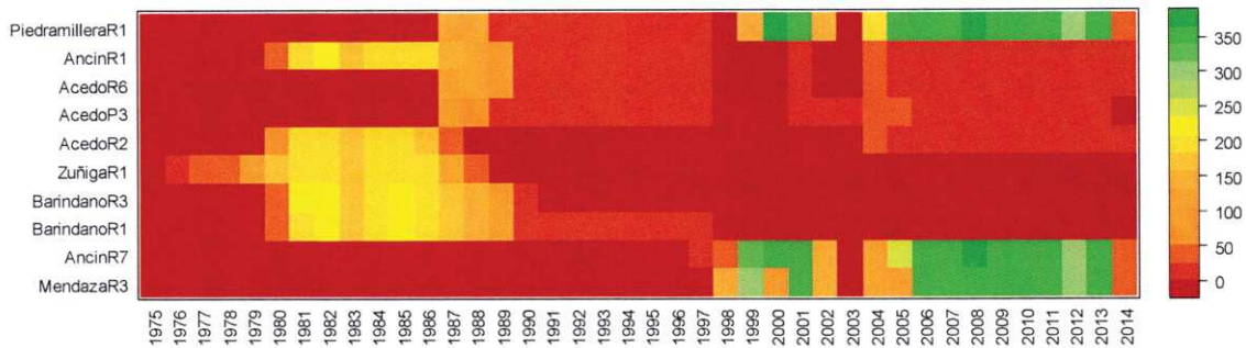
Figura 9: Número de días con datos válidos para cada año en las series de piezometría disponibles en la zona de estudio.
