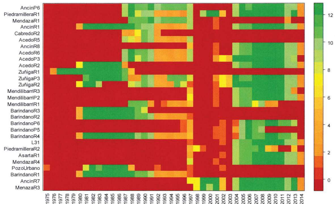
Figura 10: Número de meses con datos válidos para cada año en las series de piezometría disponibles en la zona de estudio.
