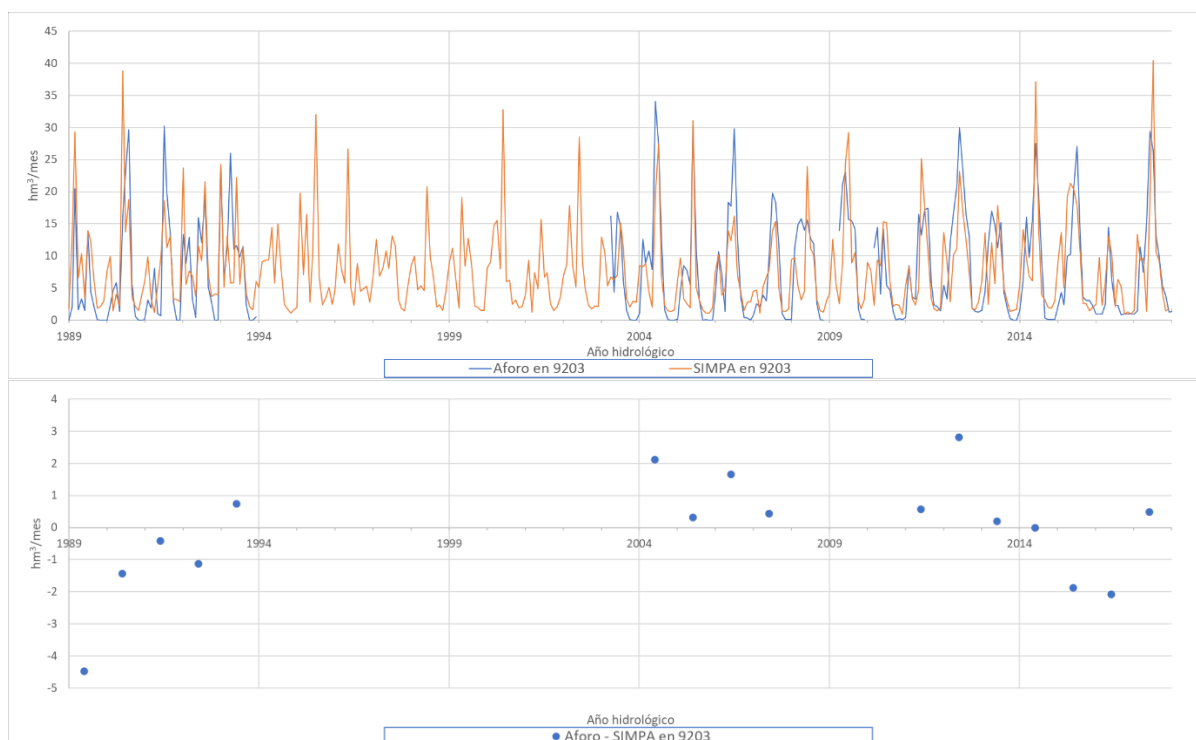
Figura 16. Comparación de la serie de aportación registrada en la estación 9203 Río Hija en Reñosa con la simulada mediante SIMPA
