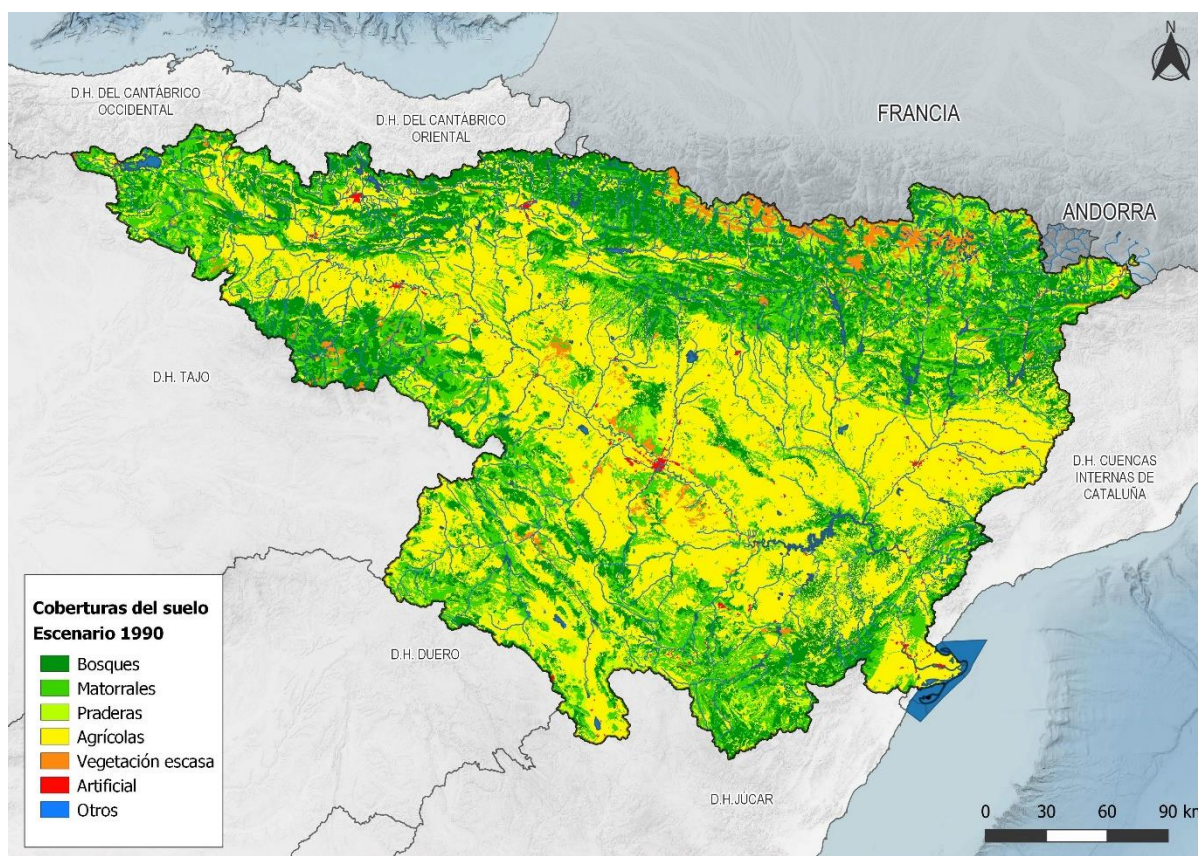
Figura 2. Mapa reclasificado de usos del suelo CLC 1990
