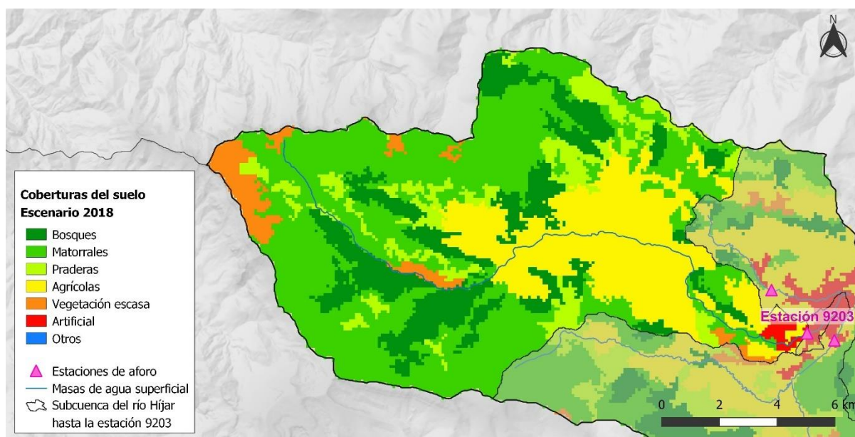
Figura 39. Usos del suelo en la subcuenca del río Híjar hasta la estación 9203 en el año 2018
