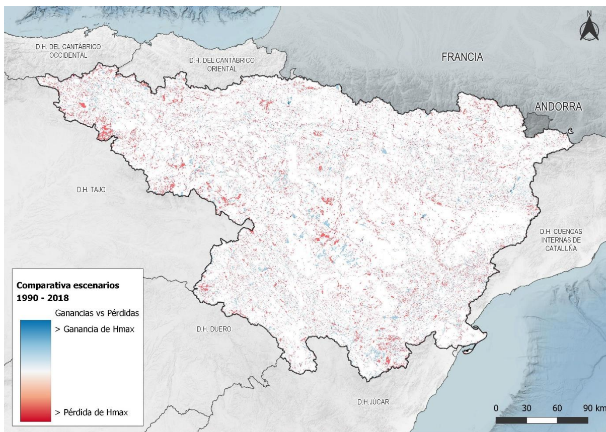
Figura 6. Mapa de cambio de H_{max} entre 1990 y 2018
