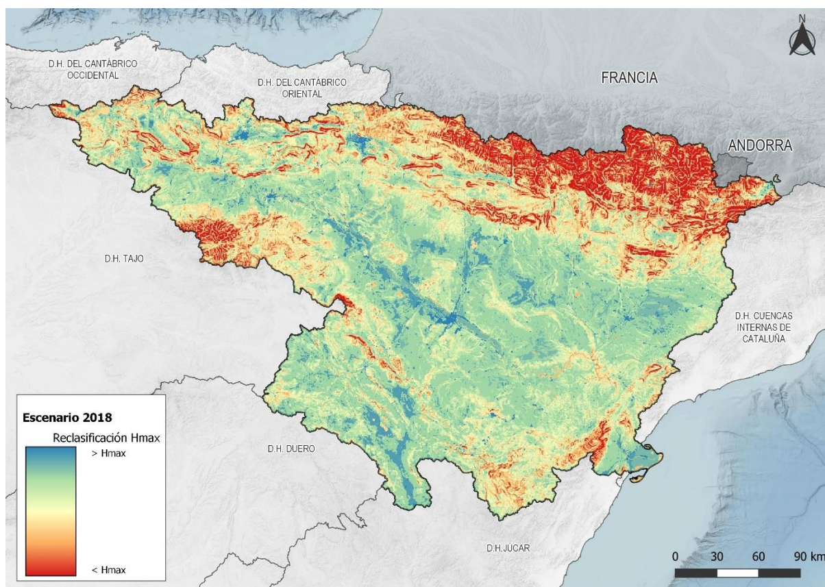
Figura 5. Mapa de H_{max} en la DHE en 2018
