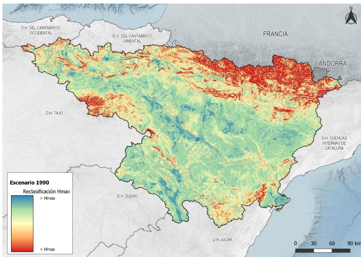
Figura 4. Mapa de H_{max} en la DHE en 1990
