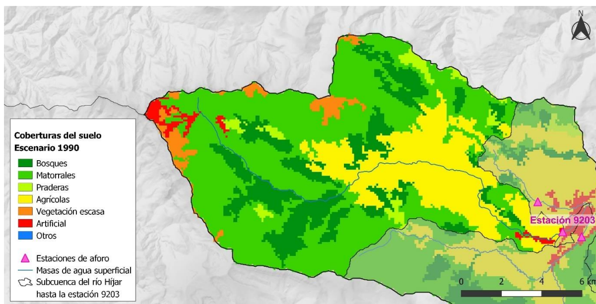
Figura 38. Usos del suelo en la subcuenca del río Híjar hasta la estación 9203 en el año 1990
