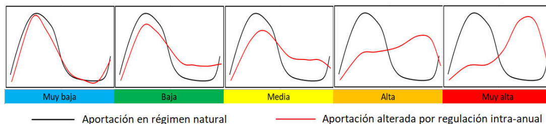
Figura 3. Visión idealizada de diferentes grados de alteración hidrológica de la modulación caudal por regulación intra-anual en embalse
