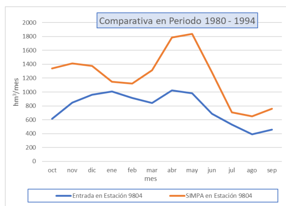
Figura 24. Comparación de la aportación media mensual de la serie de aportación entrante en 9804 Embalse Ribarroja con su aportación natural simulada mediante SIMPA (hm³/mes).
