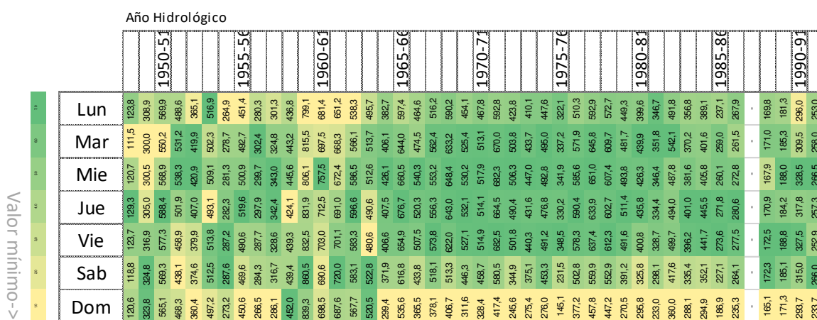
Figura 31. Análisis del caudal medio diario por año hidrológico según los días de la semana en la estación 9121 Río Ebro en Flix ( \text{m}^3/\text{s} ).
