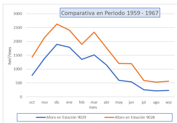
Figura 21. Comparación de las aportaciones medias mensuales de las series registradas en la estación 9029 Río Ebro en Mequinenza y 9028 Río Ebro en (hm³/mes).
