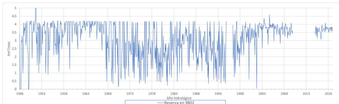
Figura 29. Variación de la reserva en 9802 Embalse Flix ( \text{hm}^3 ).
