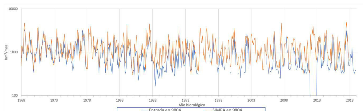
Figura 23. Comparación de la serie de aportación entrante en 9804 Embalse Ribarroja con la natural simulada mediante SIMPA (hm³/mes).
