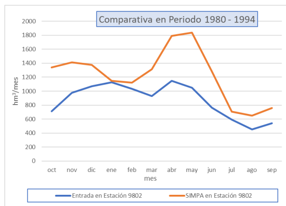
Figura 28. Comparación de la aportación media mensual entrante en 9802 Embalse Flix con su aportación natural simulada mediante SIMPA ( \text{hm}^3/\text{mes} ).
