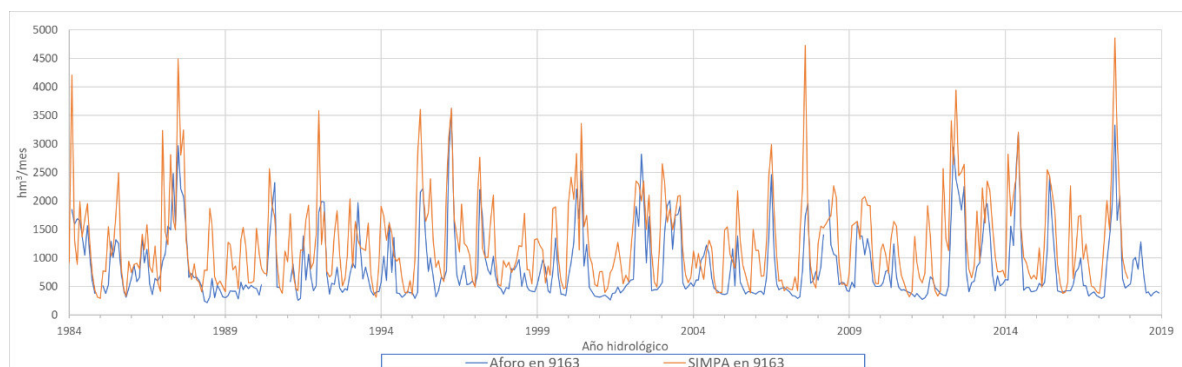
Figura 32. Comparación de la serie de aportación registrada en 9163 Río Ebro en Ascó con la natural simulada mediante SIMPA ( \text{hm}^3/\text{mes} ).
