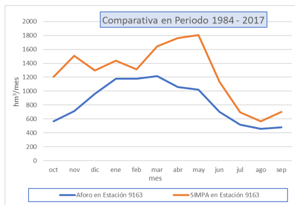
Figura 33. Comparación de la aportación media mensual de la serie registrada en la estación 9163 Río Ebro en Ascó con su aportación natural simulada mediante SIMPA ( \text{hm}^3/\text{mes} ).
