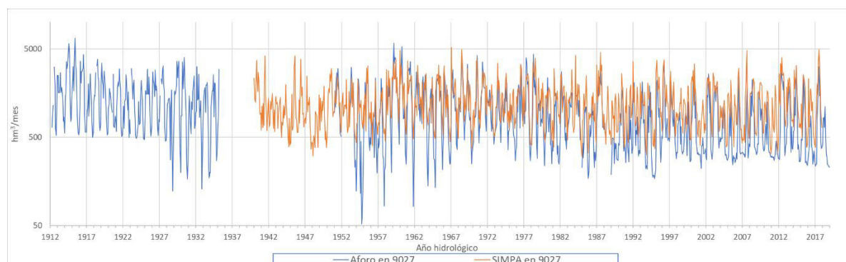
Figura 35. Comparación de la serie de aportación registrada en 9027 Río Ebro en Tortosa con la natural simulada mediante SIMPA (hm 3 /mes).
