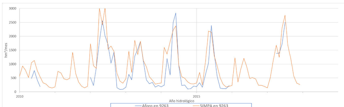
Figura 8. Comparación de la serie de aportación registrada en la estación 9263 Río Ebro en Gelsa con la natural simulada mediante SIMPA ( \text{hm}^3/\text{mes} ).
