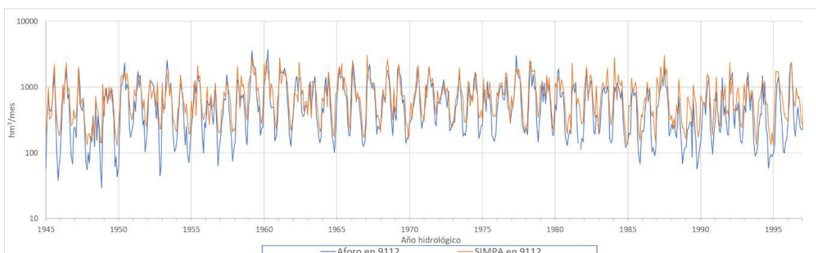
Figura 10. Comparación de la serie de aportación registrada en la estación 9112 Río Ebro en Sástago con la natural simulada mediante SIMPA ( \text{hm}^3/\text{mes} ).
