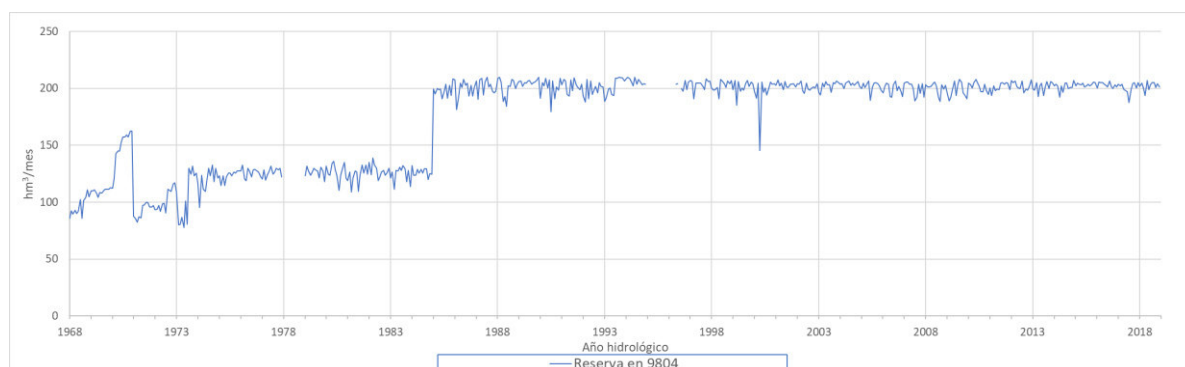
Figura 25. Variación de la reserva en 9804 Embalse Ribarroja (hm³).
