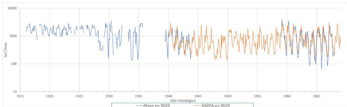
Figura 17. Comparación de la serie de aportación registrada en la estación 9029 Río Ebro en Mequinenza con la natural simulada mediante SIMPA ( \text{hm}^3/\text{mes} ).
