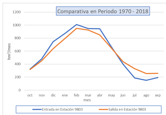
Figura 14. Comparación de la aportación media mensual entrante y saliente de 9803 Embalse Mequinenza con su aportación natural simulada mediante SIMPA ( \text{hm}^3/\text{mes} ).
