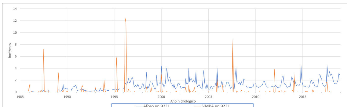
Figura 16. Comparación de la serie de aportación registrada en la estación 9231 Barranco Valcuerna en Candanos con la natural simulada mediante SIMPA ( \text{hm}^3/\text{mes} ).
