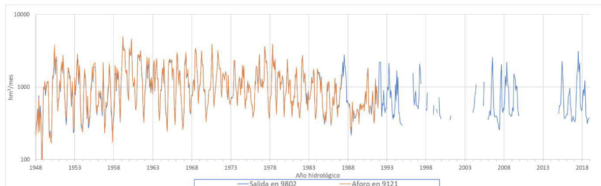
Figura 30. Comparación de la serie de aportación saliente de 9802 Embalse Flix con la aportación registrada en la estación 9121 Río Ebro en Flix ( \text{hm}^3/\text{mes} ).
