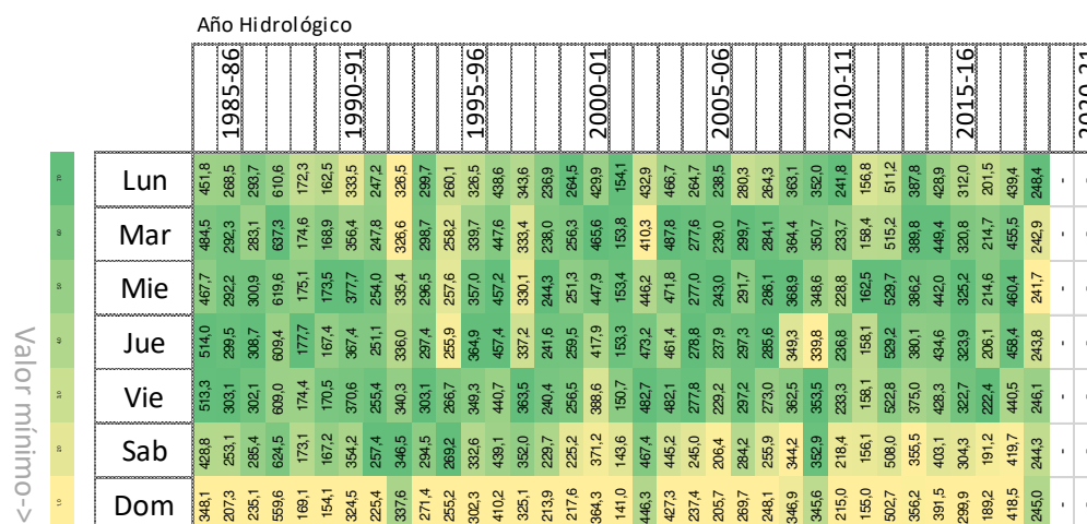
Figura 34. Análisis del caudal medio diario por año hidrológico según los días de la semana en la estación 9163 Río Ebro en Ascó (m³/s).
