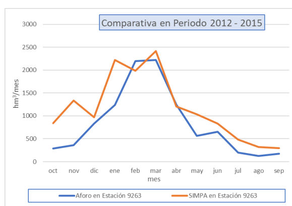
Figura 9. Comparación de la aportación media mensual de la serie registrada en la estación 9263 Río Ebro en Gelsa con su aportación natural simulada mediante SIMPA ( \text{hm}^3/\text{mes} ).
